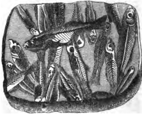
LEBIAS CEPHALOTIS. Cycloids of Aix. ( Miocene. )
